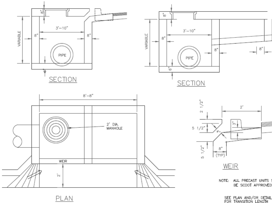
TYPE 17 CATCH BASIN N.T.S
